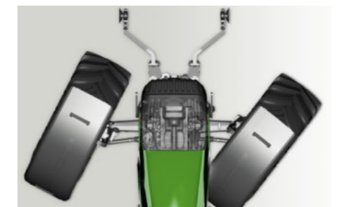
Met de VarioActive-functie leidt één keer ronddraaien van het stuur al tot de maximale stuuruitslag.
