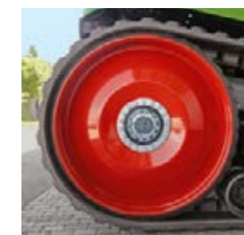
De achterste aandrijfwielen, die de rups aandrijven door middel van wrijving, brengen de kracht uitstekend over.
